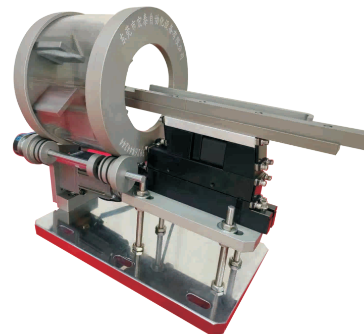
滚筒送料器
