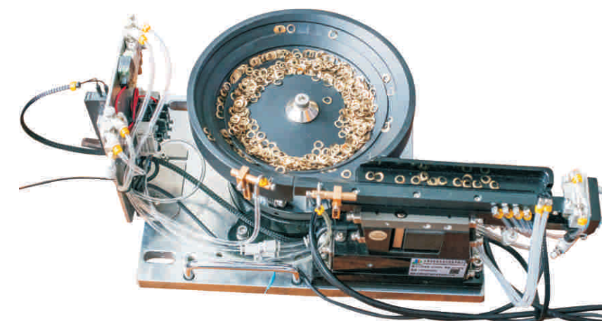
精密五金隔圈
