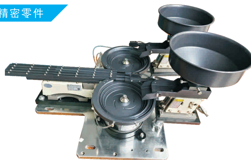
双料仓多料道精密盘
